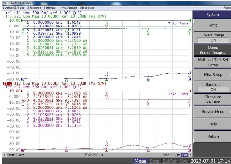
ESA-8000-70-1R 4dB
