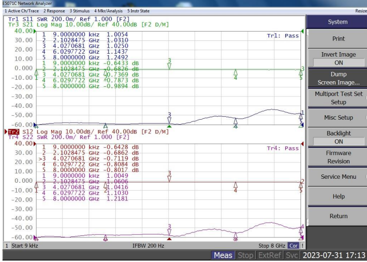
ESA-8000-70-1R 1dB
