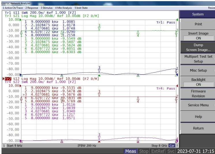
ESA-8000-70-1R 10dB
