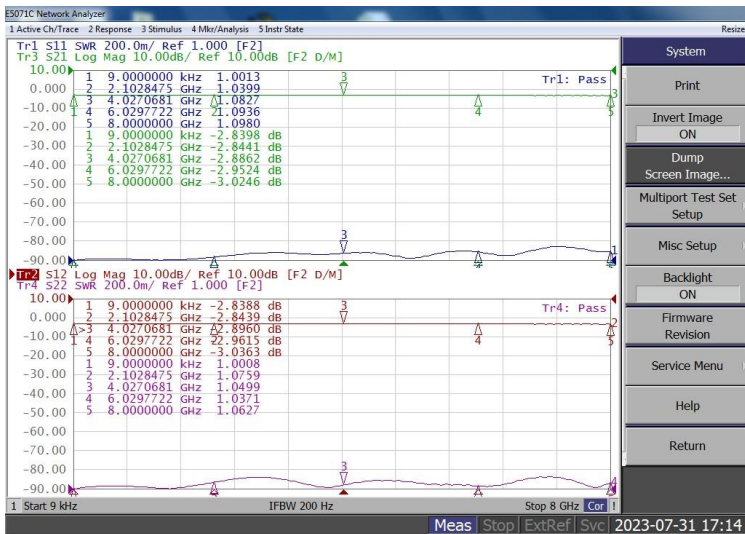
ESA-8000-70-1R 3dB
