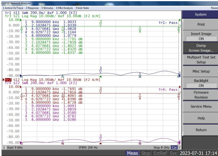
ESA-8000-70-1R 2dB
