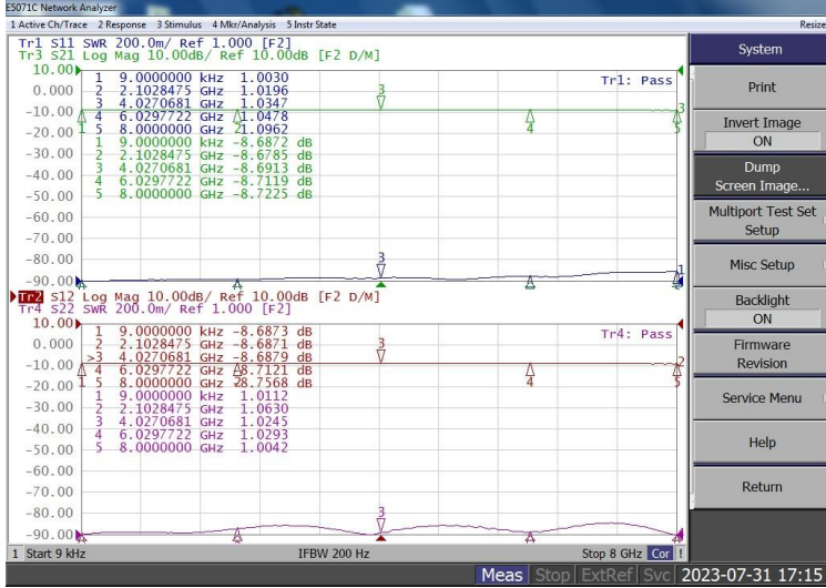
ESA-8000-70-1R 9dB
