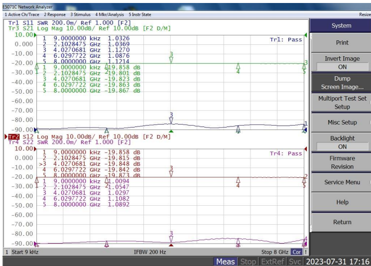
ESA-8000-70-1R 20dB
