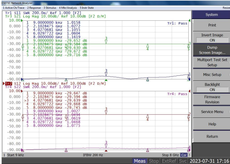
ESA-8000-70-1R 30dB
